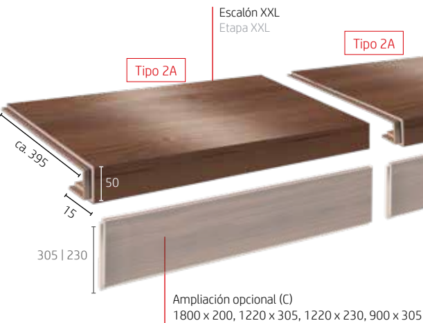
Escalera con nariz Escada com nariz
