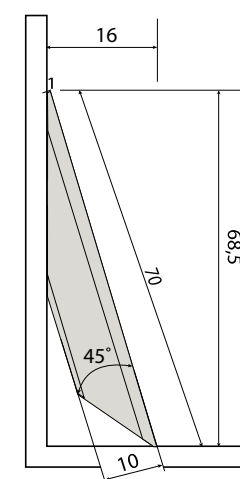
Zócalo cónico Rodapé cônico
